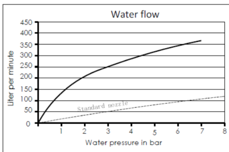
Flussdruck-Diagramm
