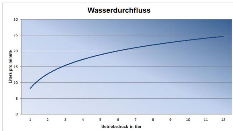
Wasserdurchfluss in L/min in Abhängigkeit vom Betriebsdruck bei Vollstrahl
