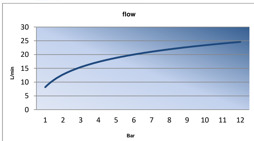
Wasserdurchfluss in l/min bei voll eingezogenem Bedienhebel, abhängig vom Druck
